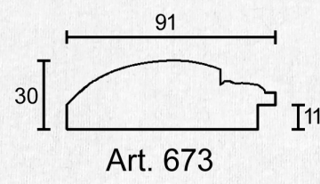
505 505R ALTA 505 R 683 505/35 658 678 681 673 682 505 R GUILL. 505/35 GUILL.
